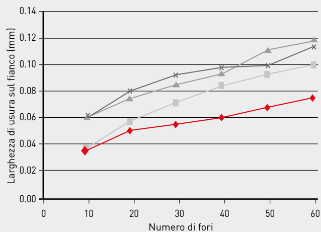
Larghezza di usura sul fianco dopo aver eseguito 60 fori
